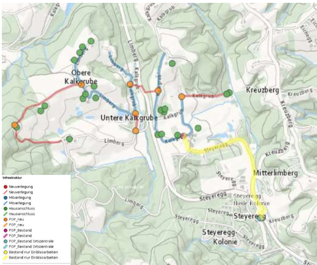
(Plandarstellung)
